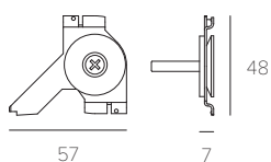
19026 Sostegno diretto
